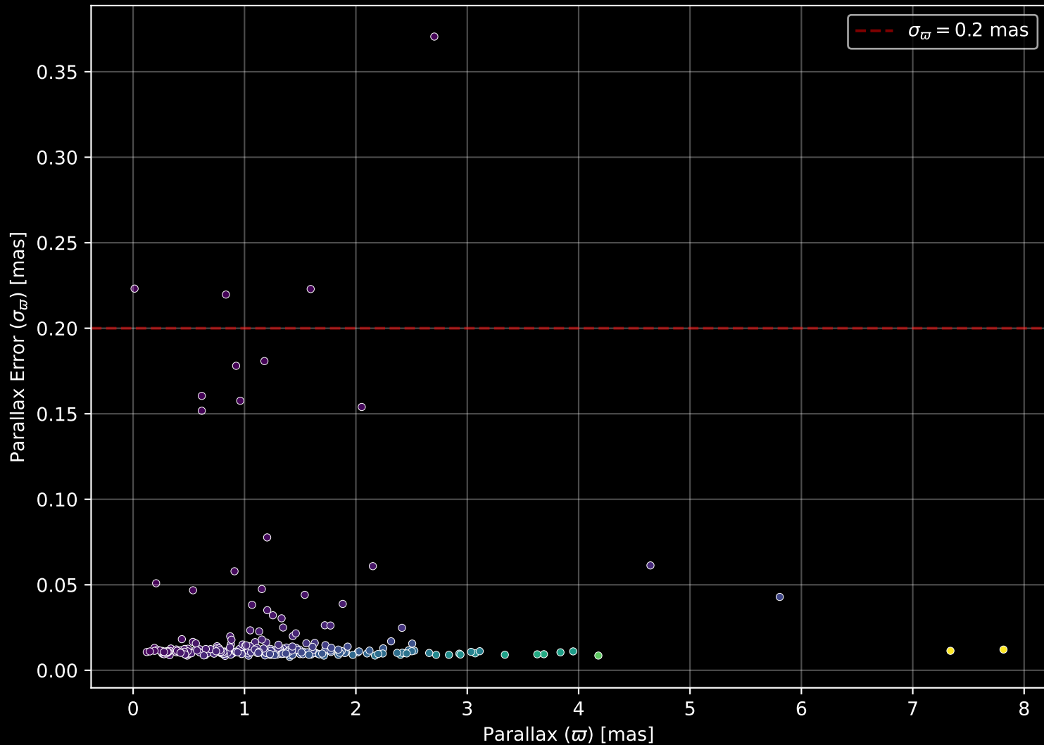
GALAH DR4 Field: [3009] Parallax Quality (n= 259)
