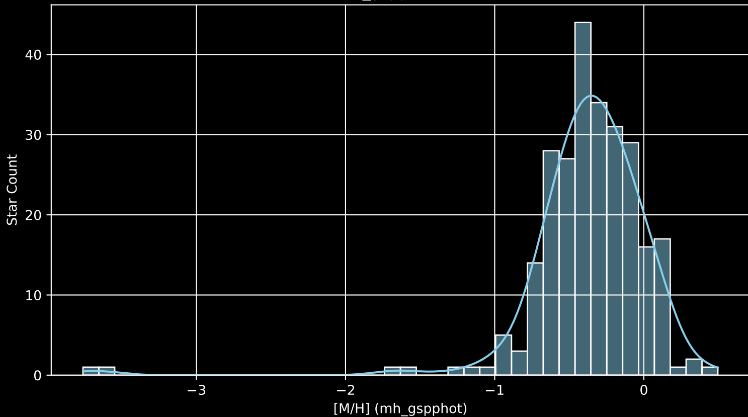
GALAH DR4 Field: [3009] [M/H] (mh_gspphot) (n= 259)
