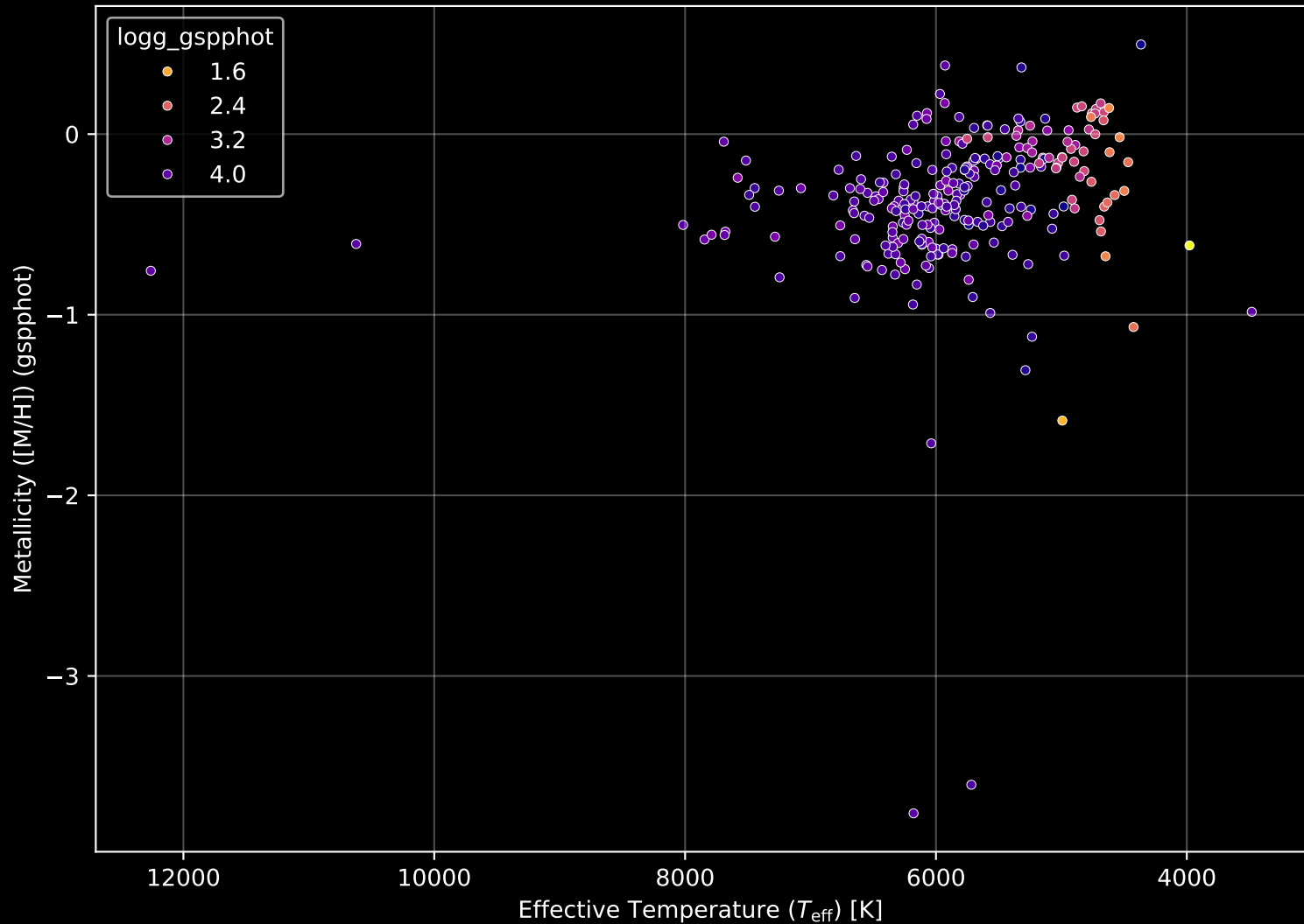
GALAH DR4 Field: [3009] Stellar Population Parameters (n= 259)
