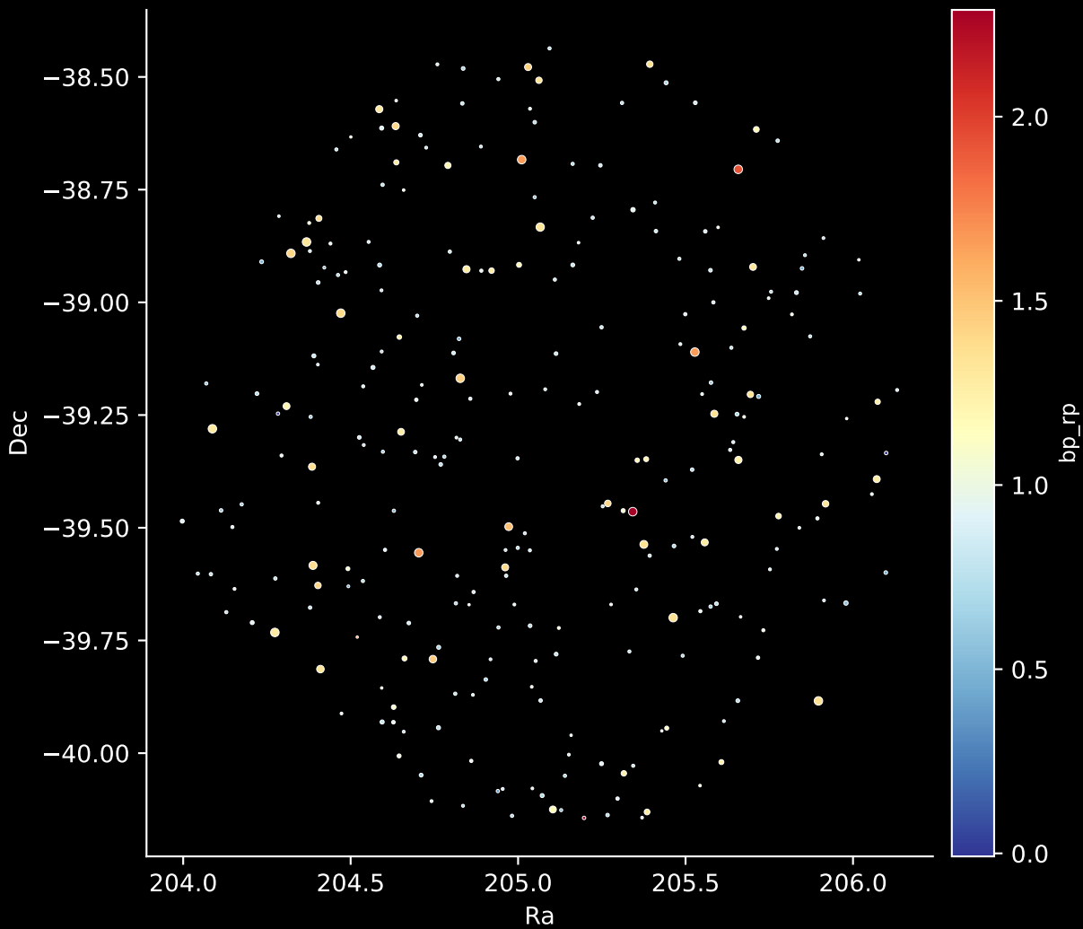
GALAH DR4 Field: [3009] Stars: 259
